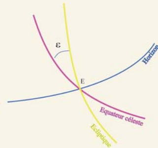
La Lune se trouve au point Est (E) sur l'horizon local au lever
