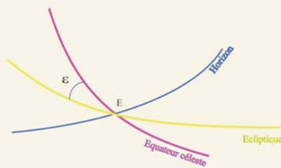
La Lune se trouve au point Est (E) sur l'horizon local au lever
