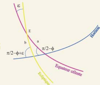
Une heure après le lever, la Lune est en E, b est la portion d'écliptique qui s'est levée sur l'horizon et a est arc horaire de 15^\circ
