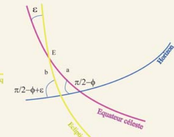
Une heure après le lever, la Lune est en E, b est la portion d'écliptique qui s'est levée sur l'horizon et a est arc horaire de 15^\circ
