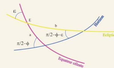
Une heure après le lever, la Lune est en E, b est la portion d'écliptique qui s'est levée sur l'horizon et a est arc horaire de 15^\circ
