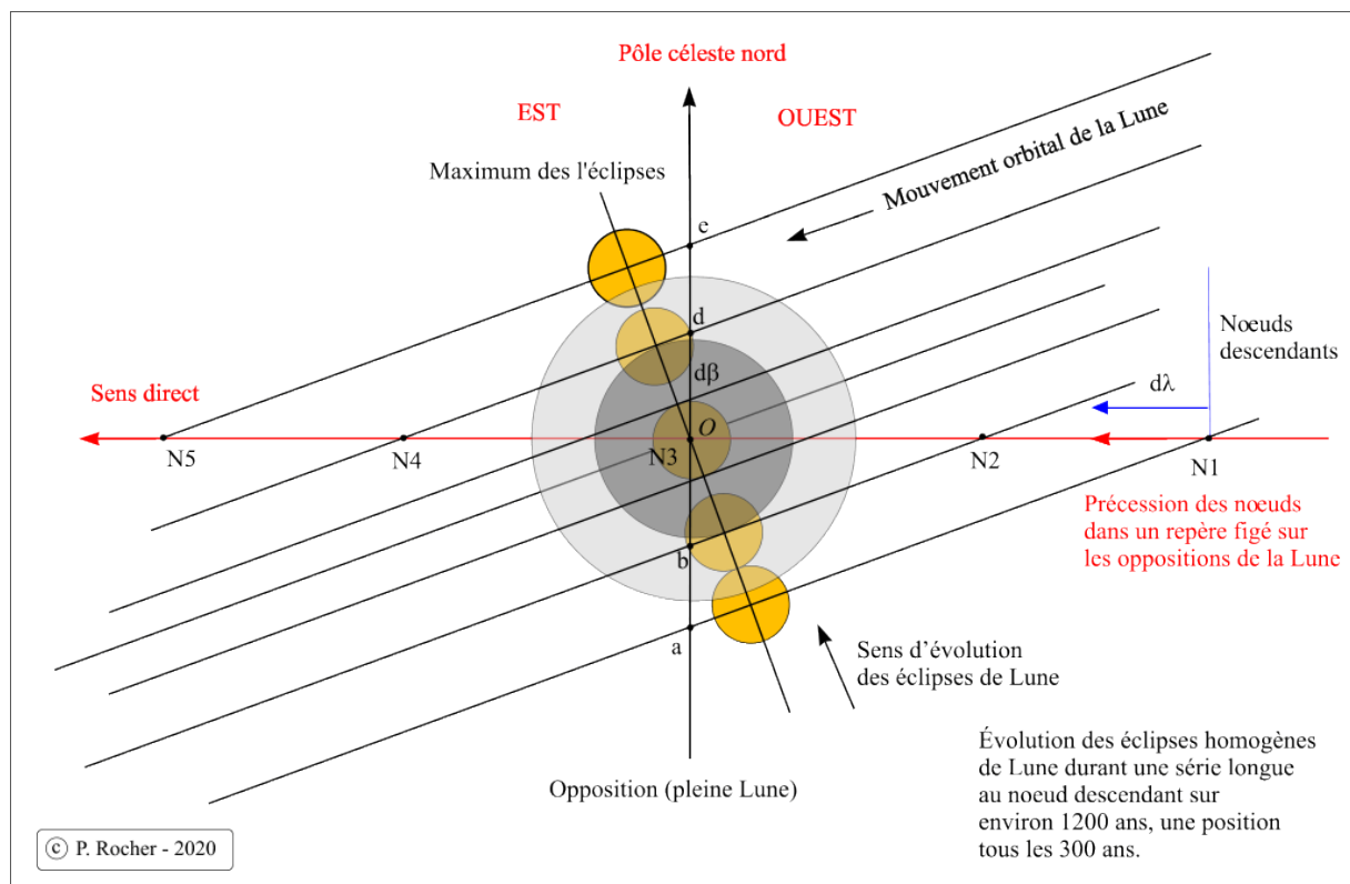
Figure 3 : Projection orthogonale de la sphère céleste éclipstique.
