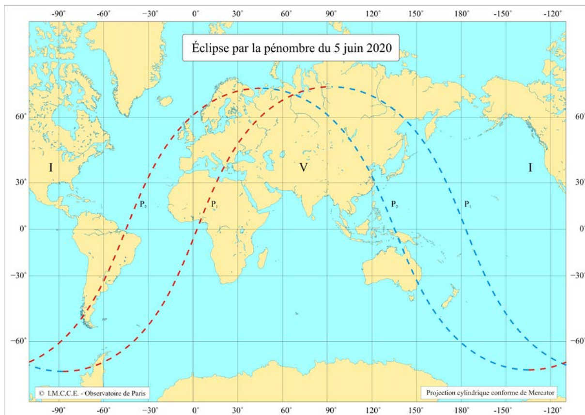
Figure 1 : Carte de l'éclipse de Lune par la pénombre du 5 juin 2020
