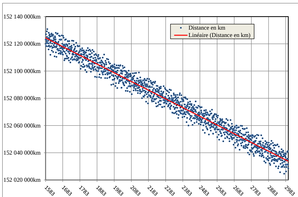
Figure 4 : Évolution des distances à l'aphélie entre 1583 et 3000.
