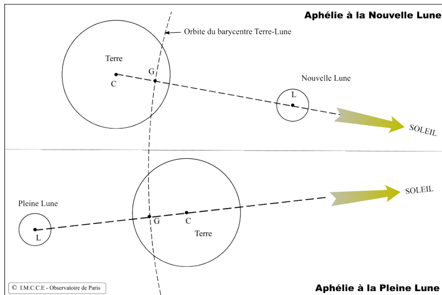
Figure 1 : Différence de distance entre deux aphélies consécutifs.
